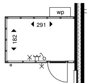
Enkele berging
