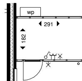
Enkele berging
